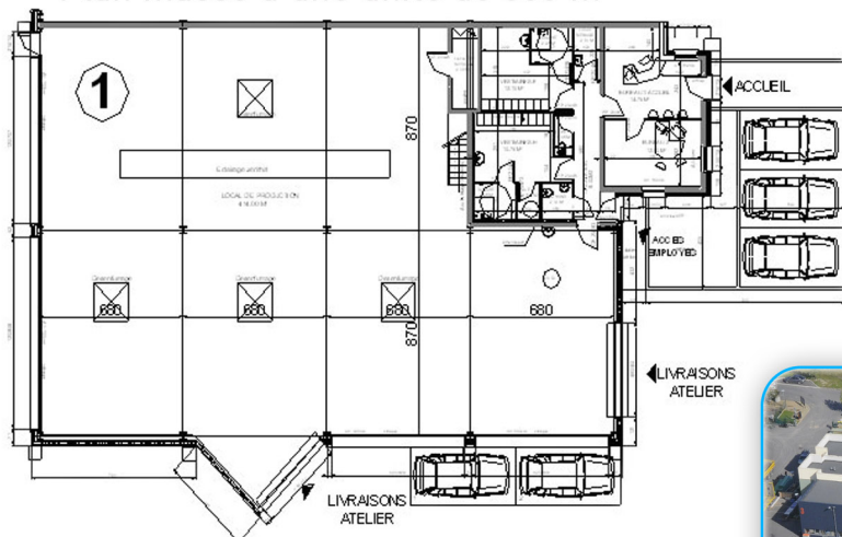
Plan masse d'une unité de 500 m 2
